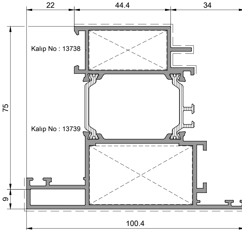
P 1184 Kanat Profili Ağırlık : 2,385kg/mt
