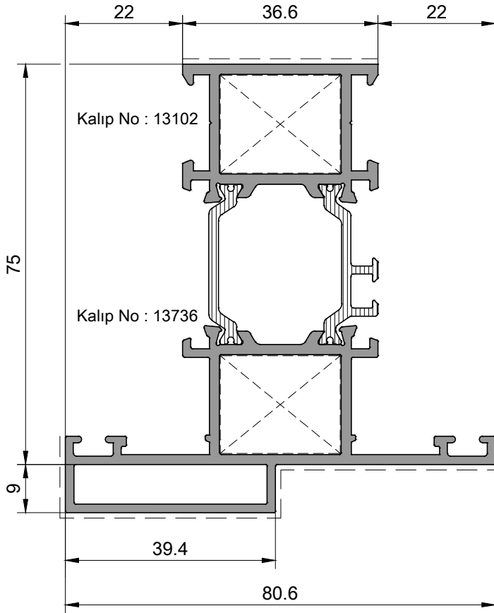
P 1181 Orta Kayıt Profili
