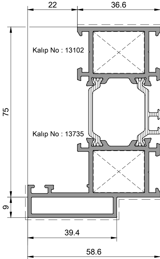
P 1182 Kasa Profili
